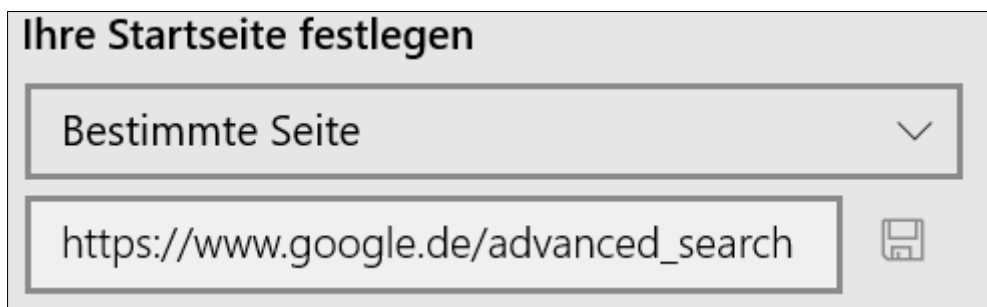
Abbildung 5: Startseite bestimmen
